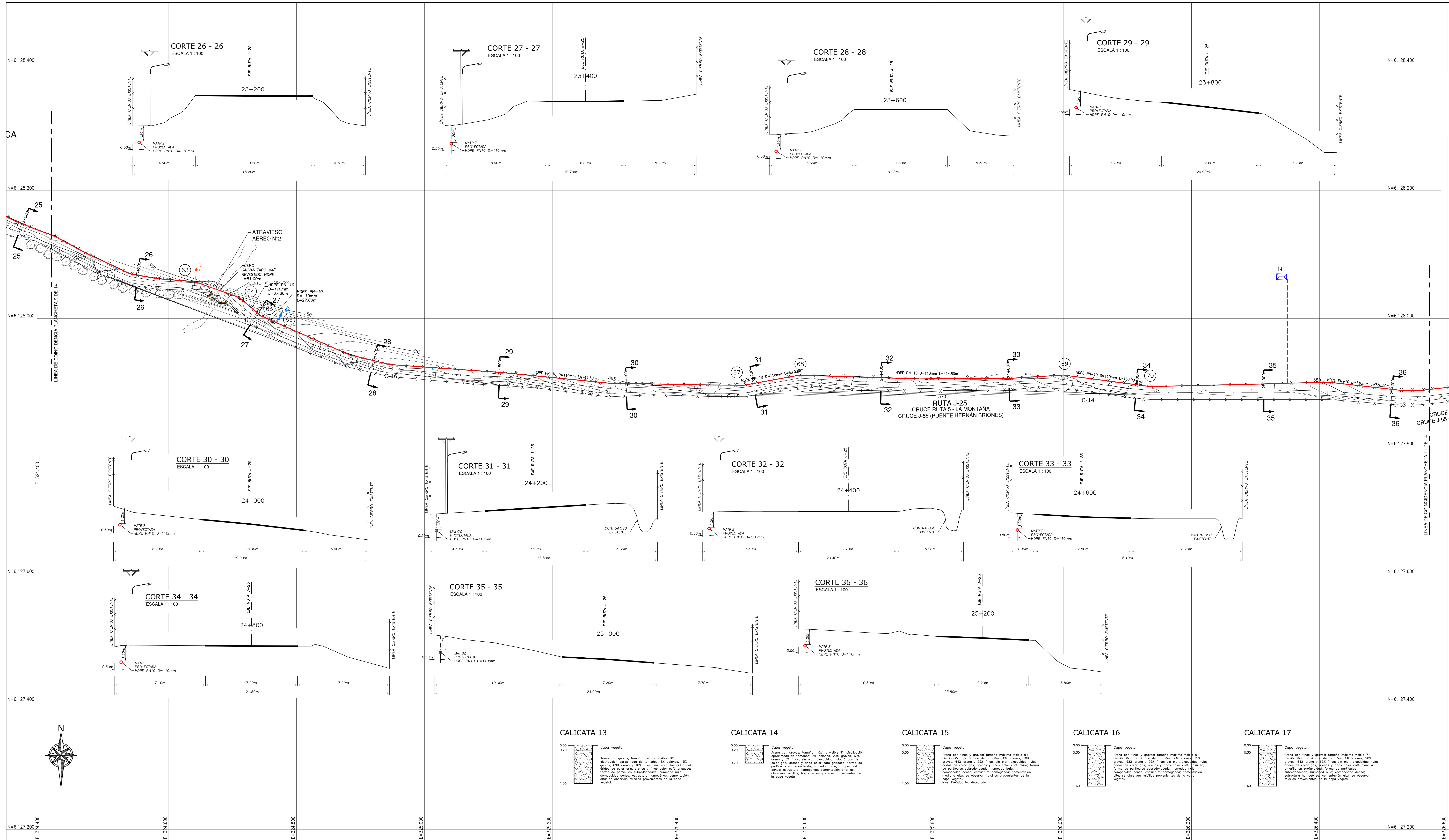
PLANTA RED PROYECTADA PLANCHETA 10 DE 14 ESCALA 1 : 2.000
